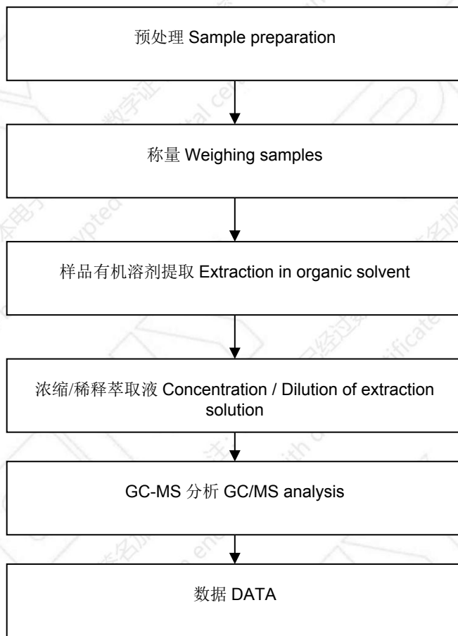
邻苯二甲酸酯类测试流程 Phthalate Flow Chart
